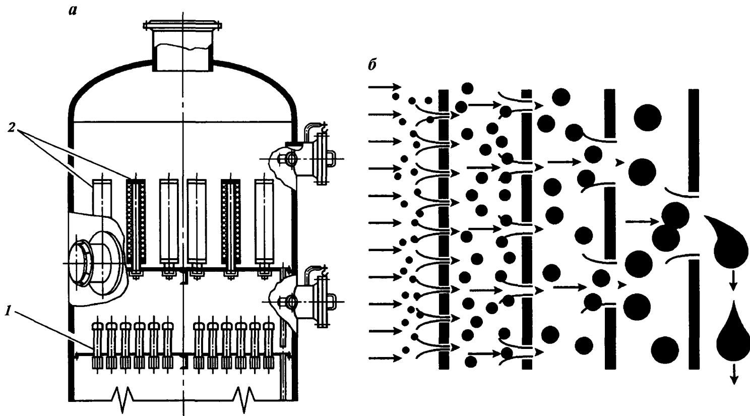
Рис. XVI-6. Схема установки фильтрующих патронов (а) и принцип действия фильтрующих патронов фирмы "Палл" (б): 1 — центробежные элементы; 2 — фильтрующие патроны
